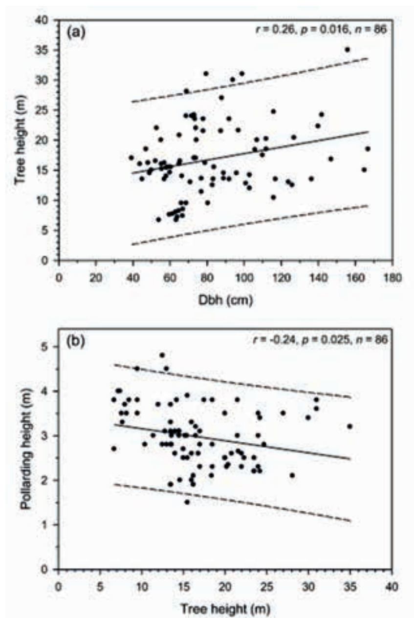
Figura 3. Principales características estructurales de los chopos cabeceros de la muestra: (a) relación positiva entre el diámetro a la altura del pecho (Dbh) y la altura del árbol, y (b) relación negativa entre la altura del árbol y la altura de la cruz. Las estadísticas correspondientes a las regresiones lineales (líneas continuas) se muestran en la esquina superior derecha de cada gráfico. Las líneas discontinuas muestran los intervalos de predicción del 95%.
