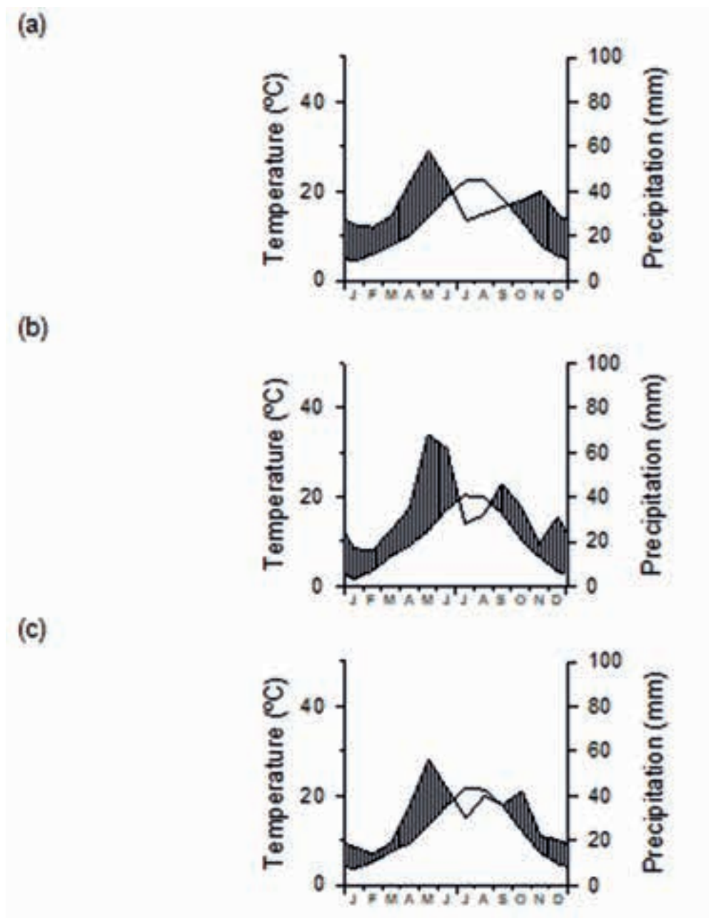
Figura S1. Diagramas climáticos de las estaciones con registros más largos en la zona de estudio: (a) Daroca ( 41^{\circ} 06' 54'' N, 1^{\circ} 25' 00'' O, 782 m s.n.m.), (b) Calamocha ( 40^{\circ} 55' 10'' N, 1^{\circ} 18' 03'' O, 884 m s.n.m.) y (c) Teruel ( 40^{\circ} 20' 38'' N, 1^{\circ} 06' 33'' O, 915 m s.n.m.).
