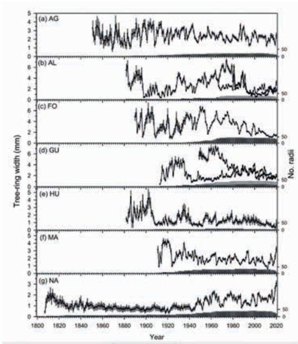
Figura 4. Datos de crecimiento de los chopos cabeceros basados en la serie media de la anchura de los anillos de los árboles calculada para cada sitio. Los datos de crecimiento se obtuvieron para testigos (barras negras) y secciones transversales de ramas (barras grises) en los sitios AL y GU. Los valores son medias \pm ES. Las barras muestran el número anual de radios medidos (ejes y derecho) con rellenos negros y grises correspondientes a los radios del tallo y de las ramas, respectivamente.
