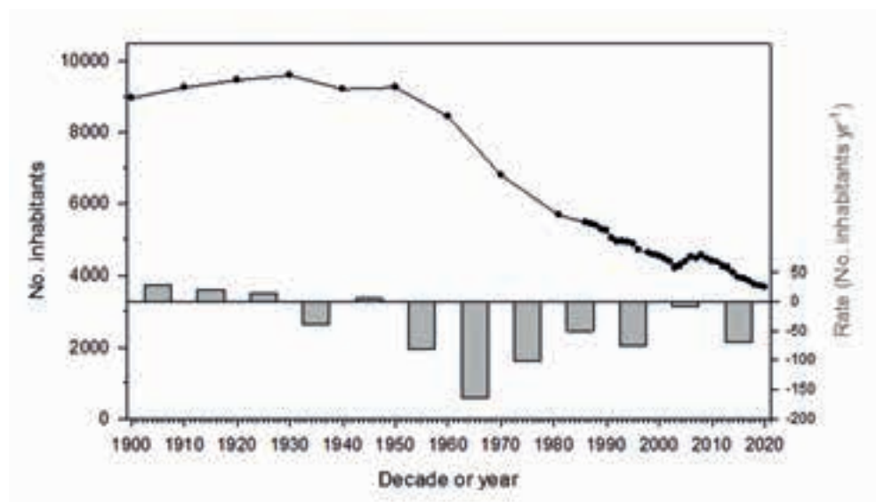
Figura S2. Cambios temporales en la población humana de la zona de estudio desde 1900 hasta 2020 basados en el número total de habitantes (línea con símbolos) y la tasa media anual de cambio calculada para cada década (barras).
