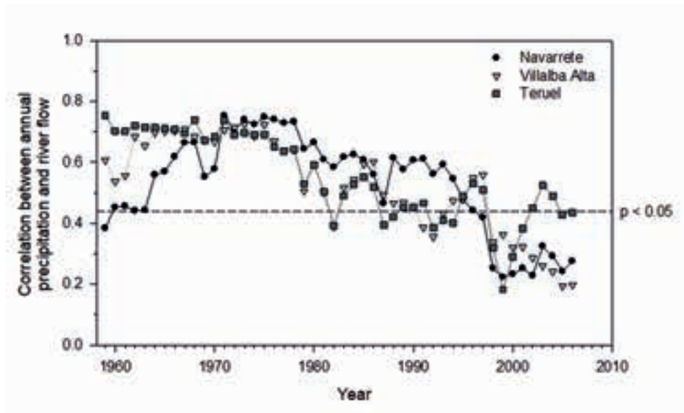
Figura S10. Correlaciones móviles calculadas relacionando la precipitación anual y el caudal del río en las tres estaciones con los datos de caudal. La línea horizontal discontinua muestra el nivel de significación de 0,05. Las correlaciones se calcularon utilizando periodos de 20 años.
