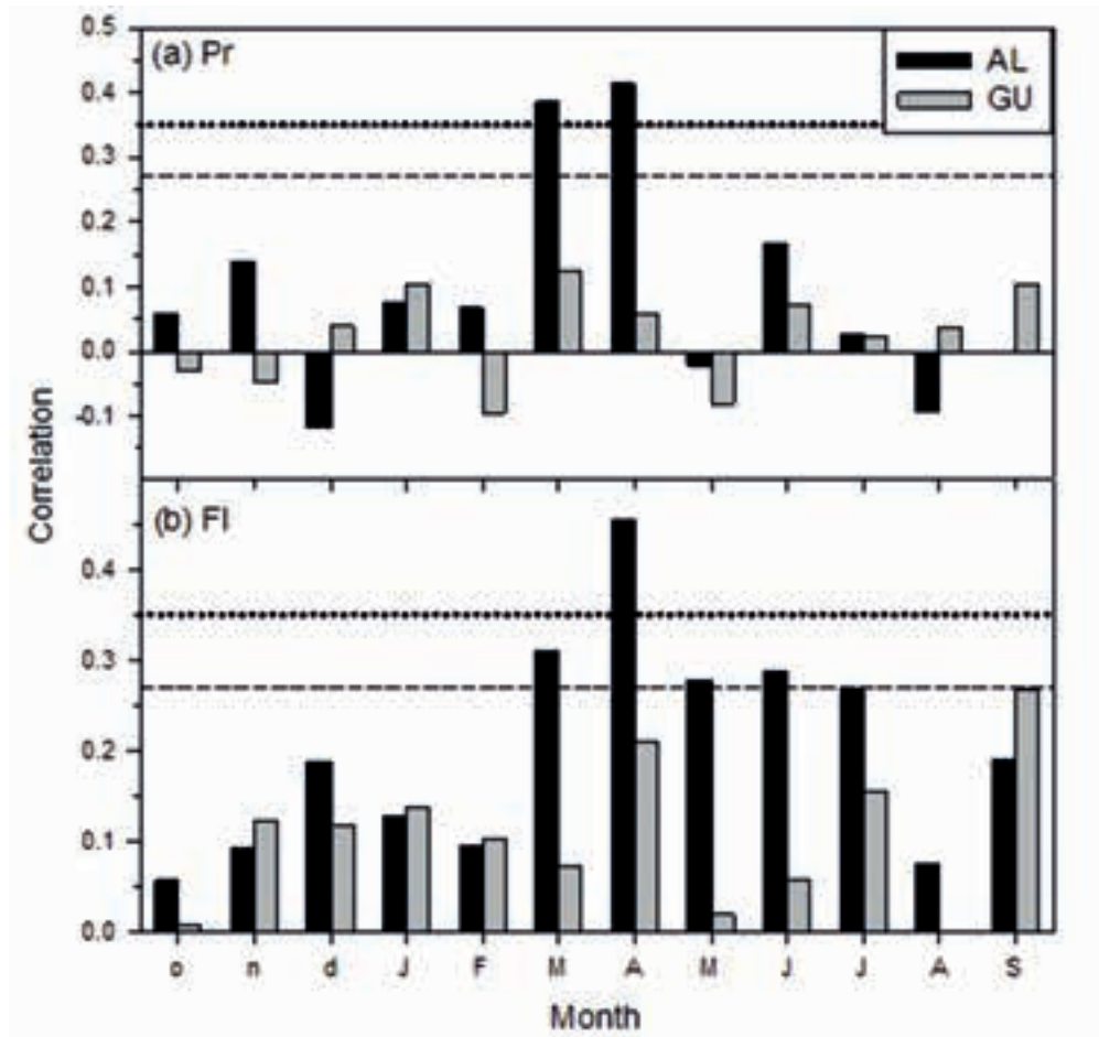
Figura S8. Correlaciones de Pearson entre los índices de crecimiento frente a la precipitación o el caudal, calculadas en los sitios de chopo cabecero donde se tomaron muestras de las ramas (sitios AL y GU). Las barras son correlaciones de Pearson obtenidas relacionando los datos de precipitación (a, Pr) o de caudal del río (b, Fl) y las series de índices de anchura de anillos medidos en las ramas. Las correlaciones se calcularon para el periodo común 1970-2020 y desde octubre anterior hasta septiembre actual. Los meses abreviados con letras minúsculas y mayúsculas corresponden a los años anterior y actual, respectivamente. Las líneas horizontales discontinuas y punteadas muestran los niveles de significación de 0,05 y 0,01, respectivamente. Los datos de caudal corresponden a la estación de Türel situada en el río Alfambra.
