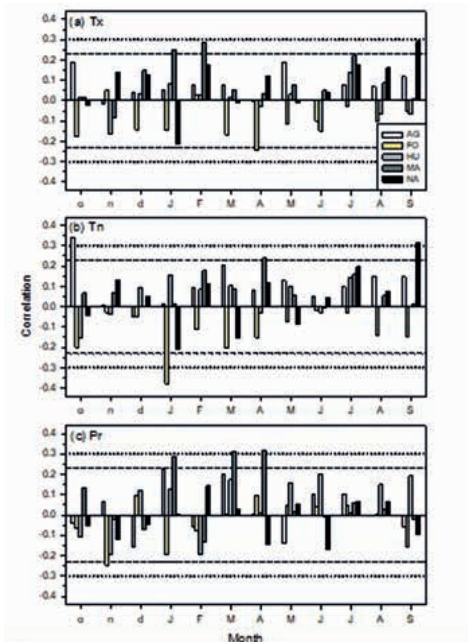
Figura S7. Correlaciones entre el clima y el crecimiento en sitios de chopo cabecero según coeficientes de Pearson (barras) calculados entre las temperaturas medias máximas (a, Tx) y mínimas (b, Tn), las precipitaciones (c, Pr) y las series de índices de anchura de anillos. Las correlaciones se calcularon para el periodo común 1950-2020 y desde octubre anterior hasta septiembre actual. Los meses abreviados con letras minúsculas y mayúsculas corresponden a los años previo y actual, respectivamente. Las líneas horizontales discontinuas y de puntos muestran los niveles de significación de 0,05 y 0,01, respectivamente.
