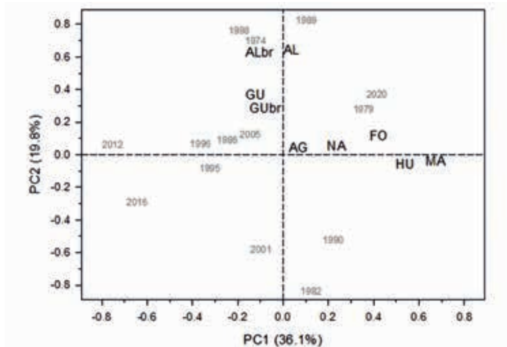
Figura S6. Diagrama de dispersión (“biplot”) que muestra las posiciones relativas de los sitios (símbolos negros) y de los años (símbolos grises) en los componentes principales primero (PC1) y segundo (PC2) de un Análisis de Componentes Principales (ACP). El ACP se calculó sobre la matriz de covarianza de las cronologías residuales de la anchura de los anillos para el periodo común 1970-2020. La varianza de cada componente se muestra entre paréntesis. Sólo se han representado los años con puntuaciones extremas de PC1 y PC2. Véanse los códigos de los sitios en las Tablas 1 y 2.
