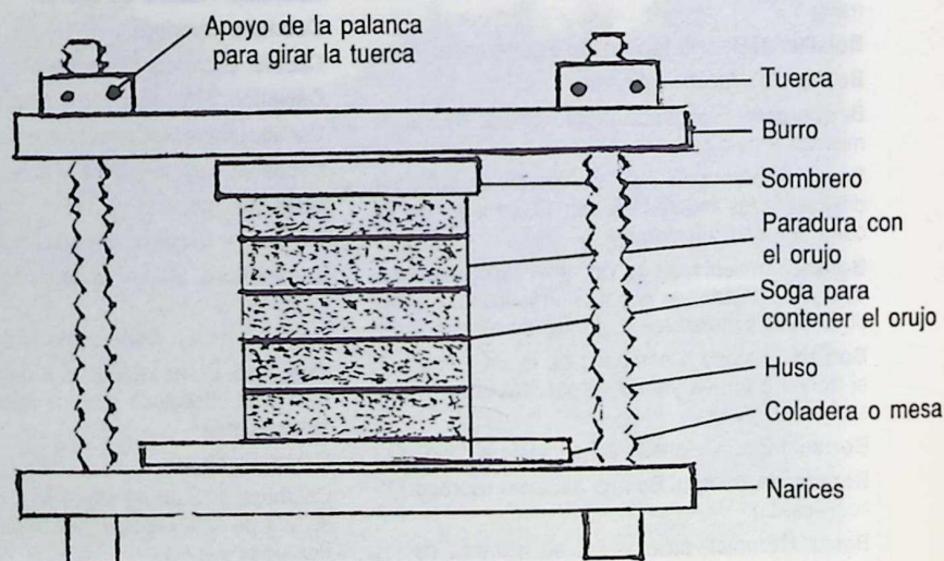
Fig. 5. Prensa Antigua de Madera. (Esquema).
