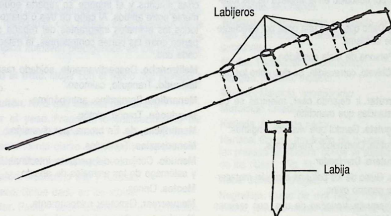
Fig. 12. Timón del Arado Romano.
