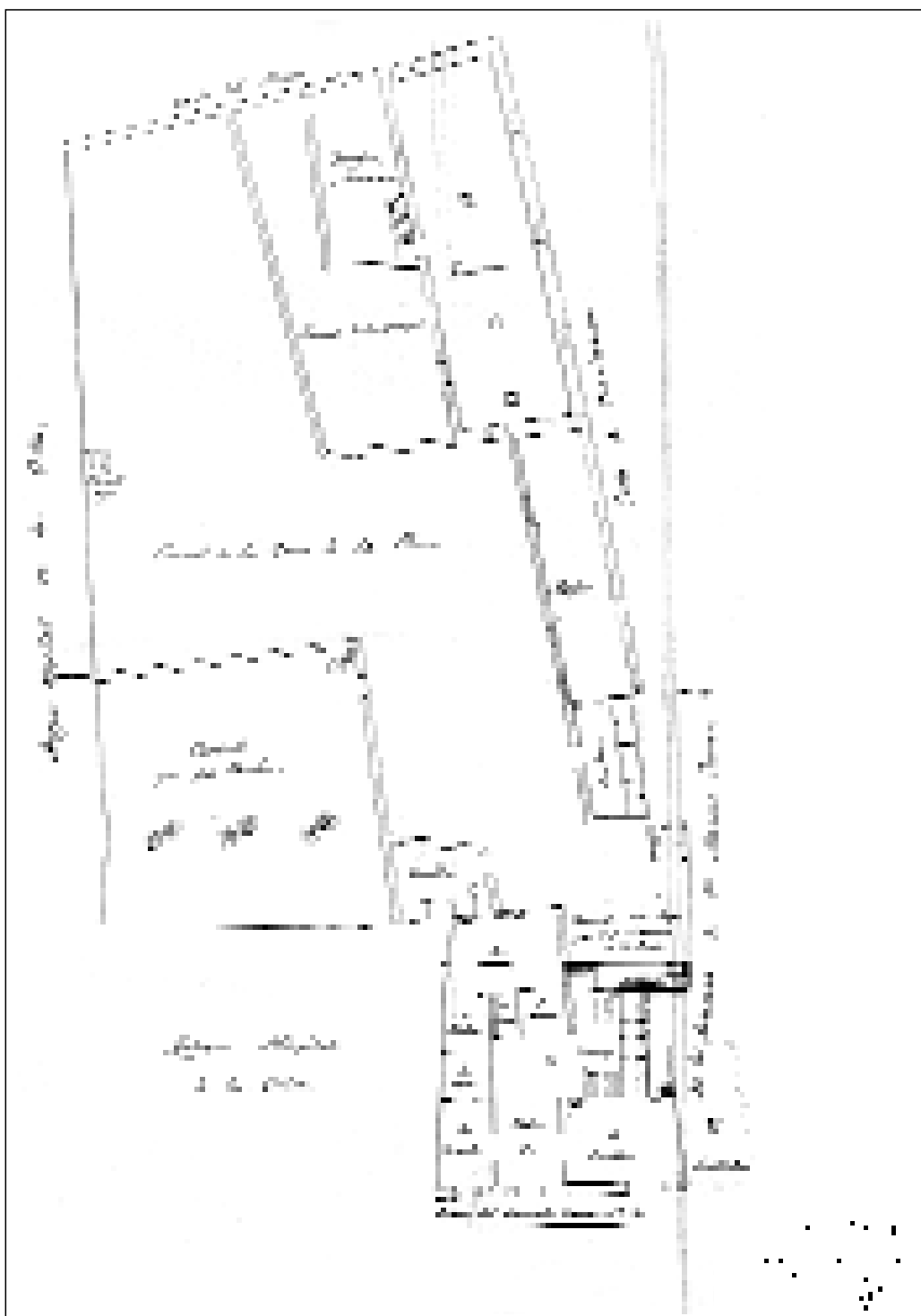
Plano que manifiesta la planta del piso bajo de la casa y demás agregados que D. Juan Almor, del comercio de esta ciudad, posee en la Villa de Egea de los Caballeros, sita en la Plaza del Mercado, señalada con el n° 2: formado a instancia del mismo Sr. Almor = Todo lo que es la casa letra A, tiene bodega, lo demás es terreno firme = la parte B, en el piso bajo y pral. es de la casa contigua n° 1 de los herederos de D. Manuel Garcés: y en el 2° piso o granero es de D. Juan Almor.
