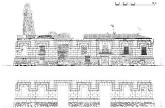
Palacio barroco inconcluso de Used. Fachada Sureste (Principal): Alzado actual y original del primer piso, único concluido. Destaca la disposición de las dos grandes puertas, que sin embargo no encajan completamente con la descripción de Fray Pedro José de Parras, así como la proporción áurea de los vanos.
